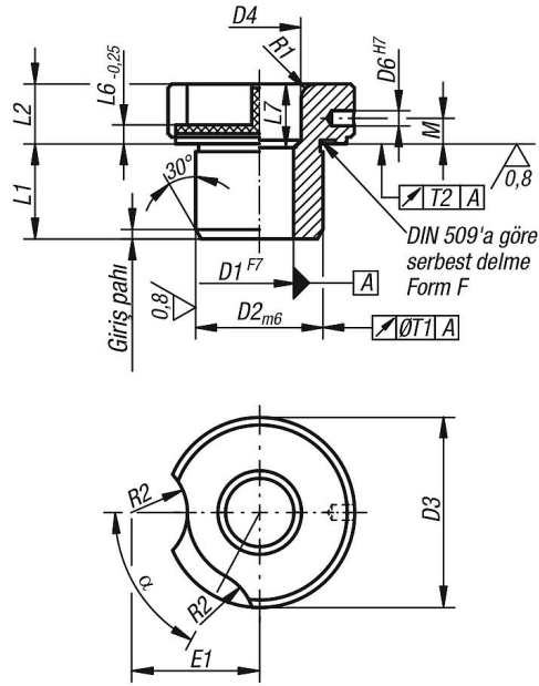
Form K Sağ dişli sağdan kesen aletler için hızlı değiştirilebilir burç
