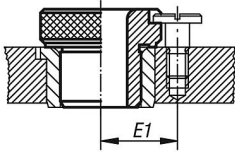
Değiştirilebilir burç, Form L DIN 172 uyarınca bilezikli delme burçlu veya DIN 179 uyarınca delme burçlu
