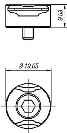
Sıkıştırma tırnağı
