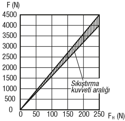
Kuvvet diyagramı
