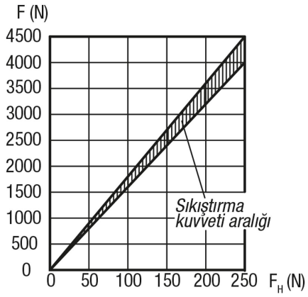
Kuvvet diyagramı
