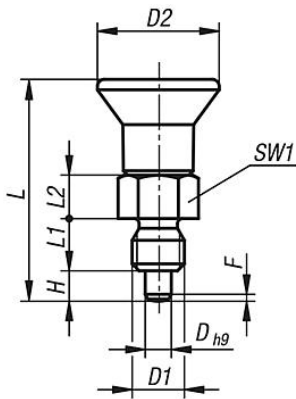
Form A kilitleme kanalsız kontra somunsuz
