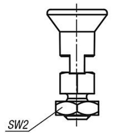
Form D kilitleme kanallı kontra somunlu
