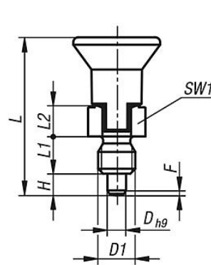
Form C kilitleme kanallı kontra somunsuz
