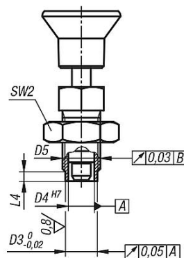
Form B ohne Rastnut mit Kontermutter
