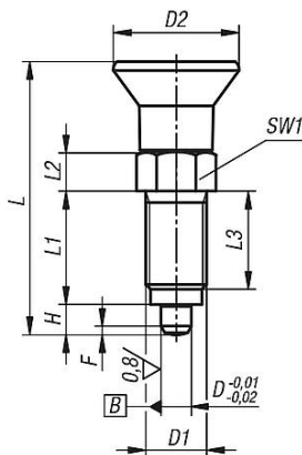
Form A ohne Rastnut ohne Kontermutter
